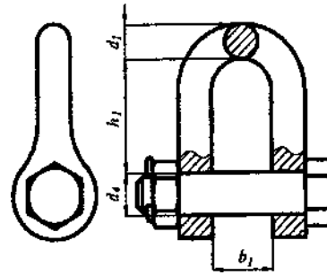
Скоба такелажная без замка
