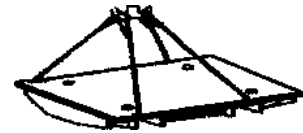
Схема строповки рамы тележки
